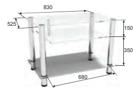
ТУМБА ПОД TV TV AS-1.1
