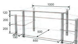
ТУМБА ПОД TV TV AS-9 (плазма)
